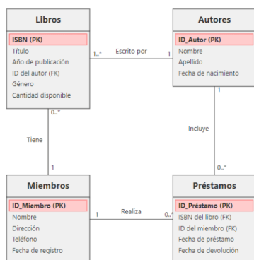
Diseño - Entidad-relación
